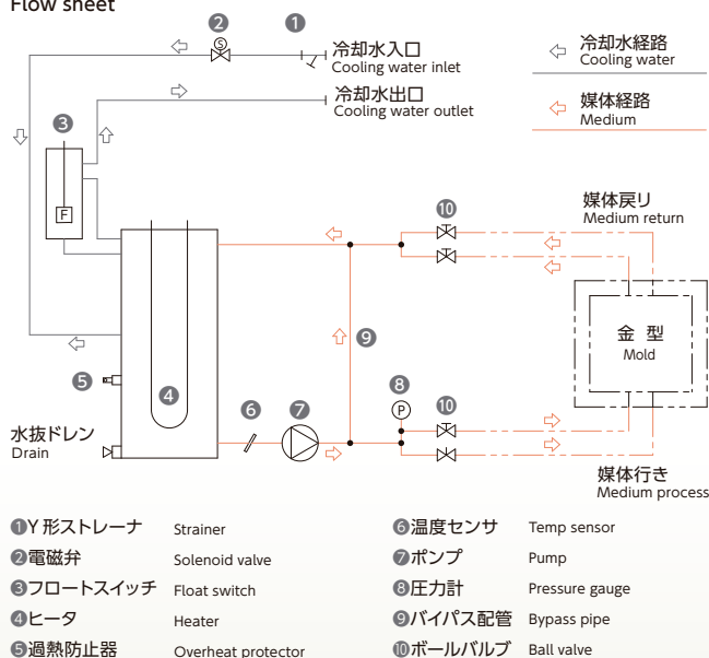
フロー図 Flow sheet
