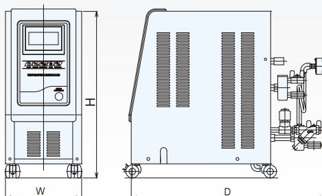
外形寸法図 Dimensions
