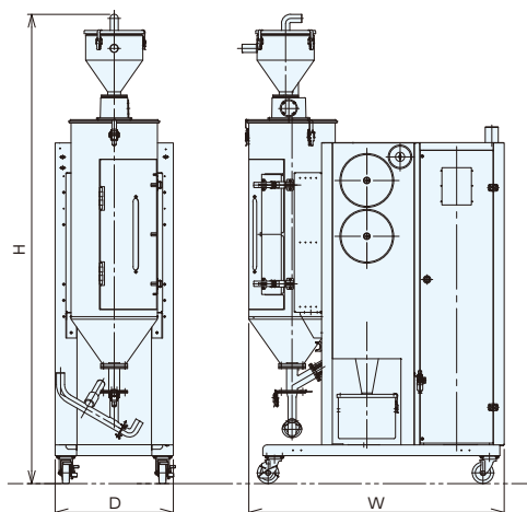
寸法表 Dimensions
