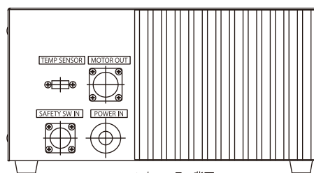
コントローラ背面
